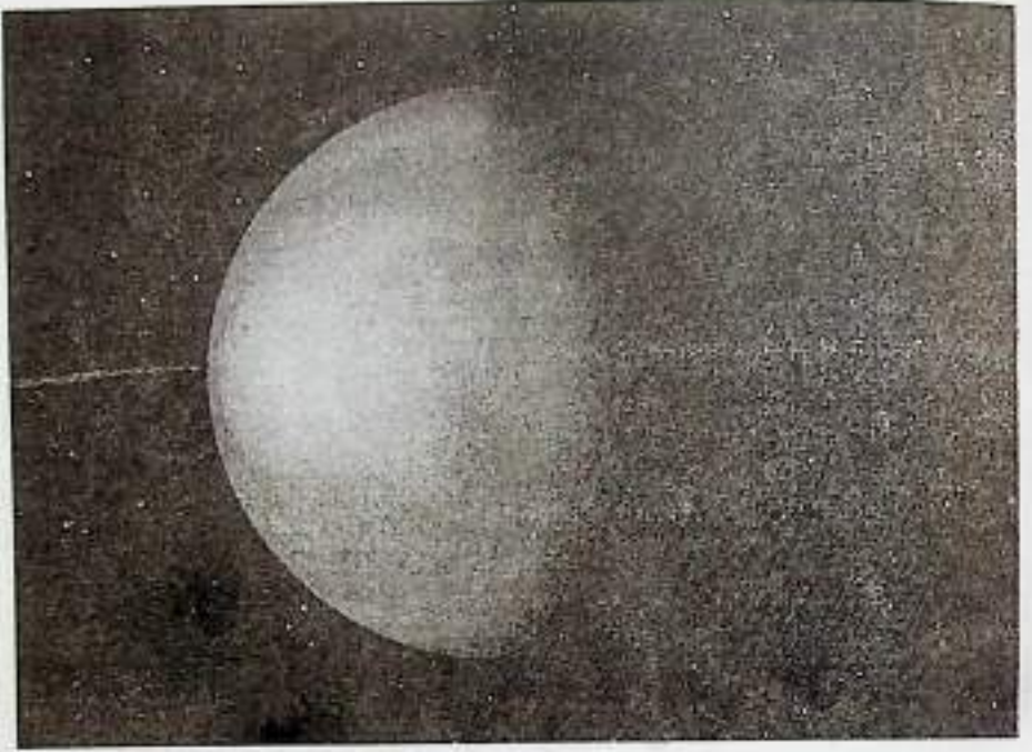
चित्रम्-१७ : शुक्रः
