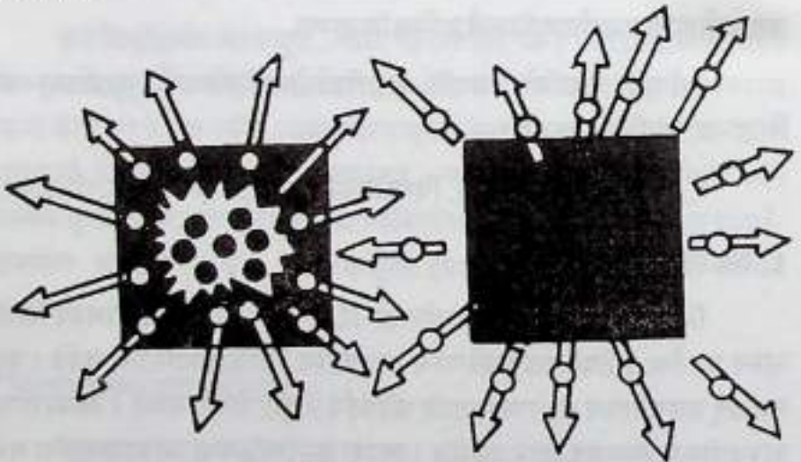
चित्रम्-४ : विस्फोटकसिद्धान्तः
