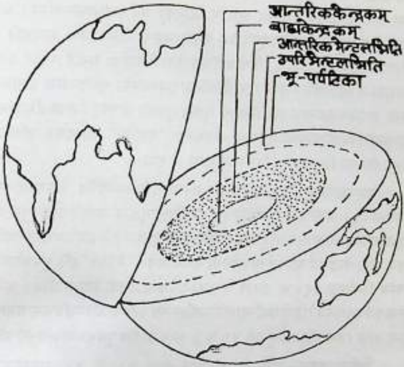
चित्रम्-४० : भूमेरान्तरिकसंरचना
