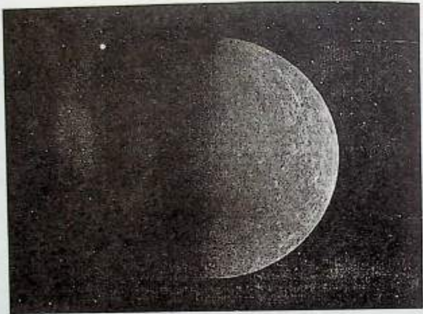
चित्रम्-१६ : बुधः
