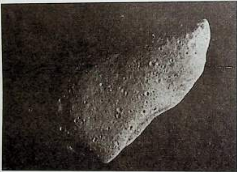
चित्रम्-३० : उल्काखण्डम्
