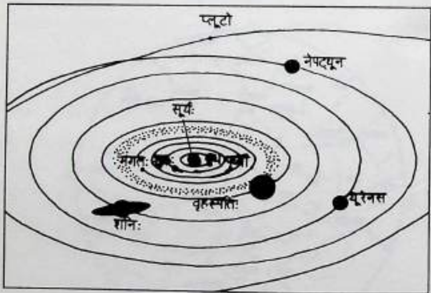
चित्रम्-९ : सौर-परिवारः
